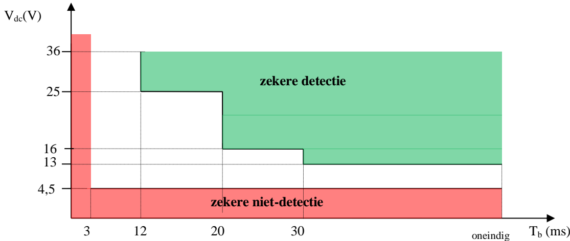
Figuur 4: Detectiezone
